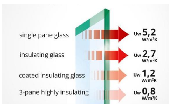
Նկար 21. Տարբեր տեսակի պատուհանների U-արժեքները:
