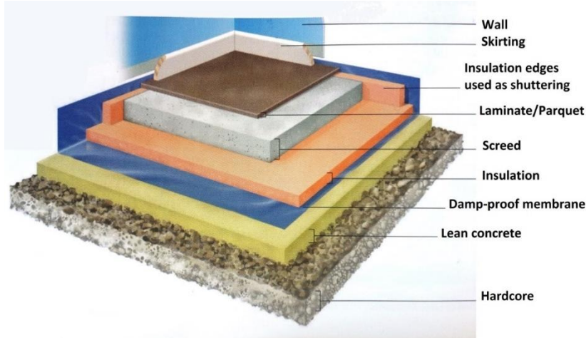
Նկար 26. Հատակի ջերմամեկուսացման սխեման:
