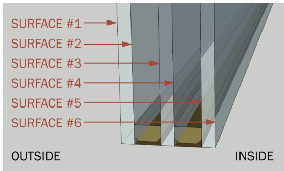
Նկար 23. Մակերևույթների համարակալումը:
