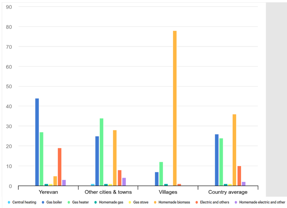
Նկար 3. Հայաստանի տնային տնտեսություններում կիրառվող ջեռուցման տեխնոլոգիաների էներգիայի ծախսը:
