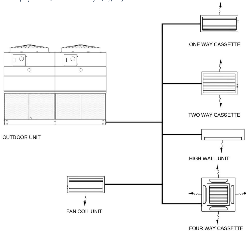
Նկար 38. ՍՓՀ համակարգի սխեման:
