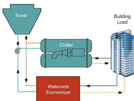
Figure 44. Ջրով աշխատող սովորական էկոնոմիզատորի դիագրամ:
