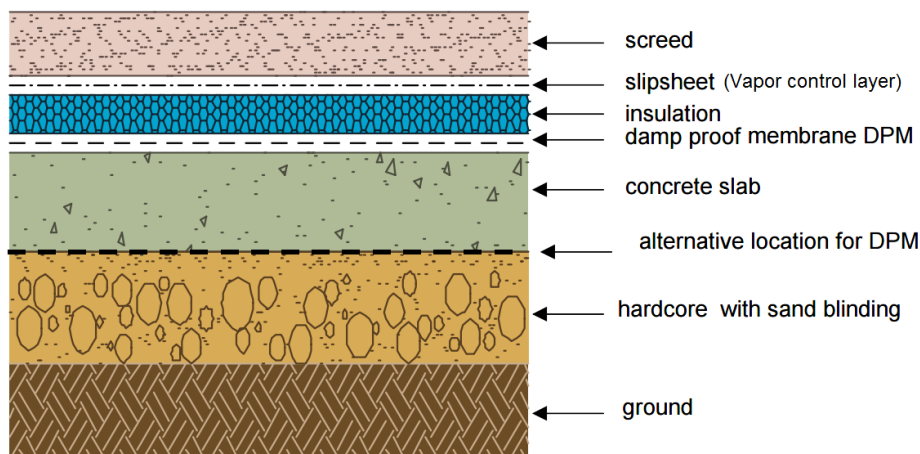
Նկար 27. Հատակի ջերմամեկուսացման այլընտրանքային սխեմա: .
