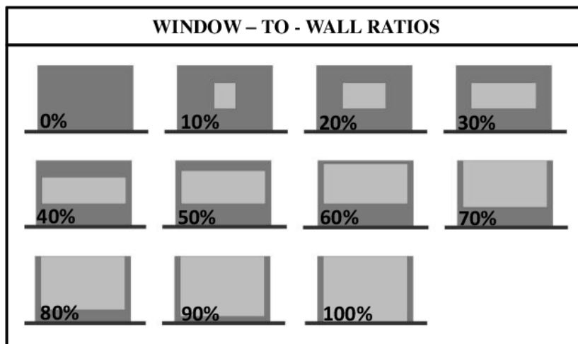
Նկար 18. Տարբեր ՊՊՀ-ն ունեցող ճակատների օրինակներ:
